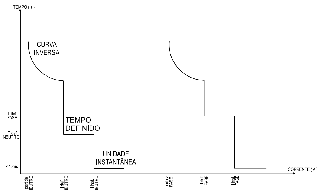
Figura 7: Curva de operação genérica
